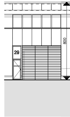
Façade Nord 1:200
